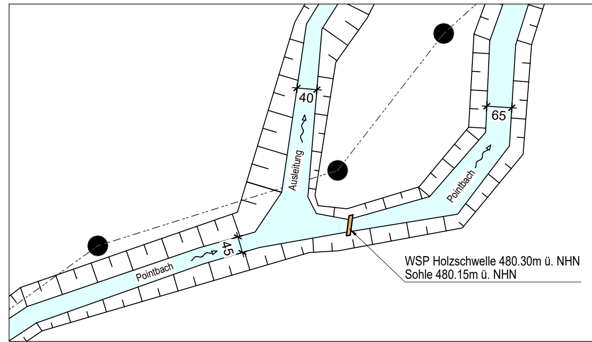
Detail 1 Ausleitungsstelle M1:100
